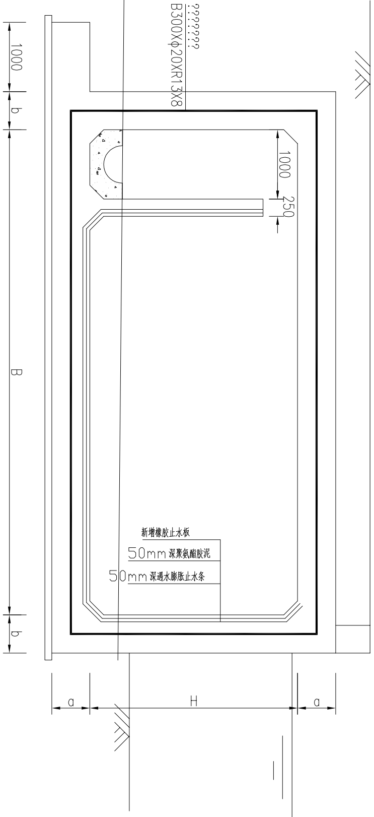
箱涵沉降缝止水断面
